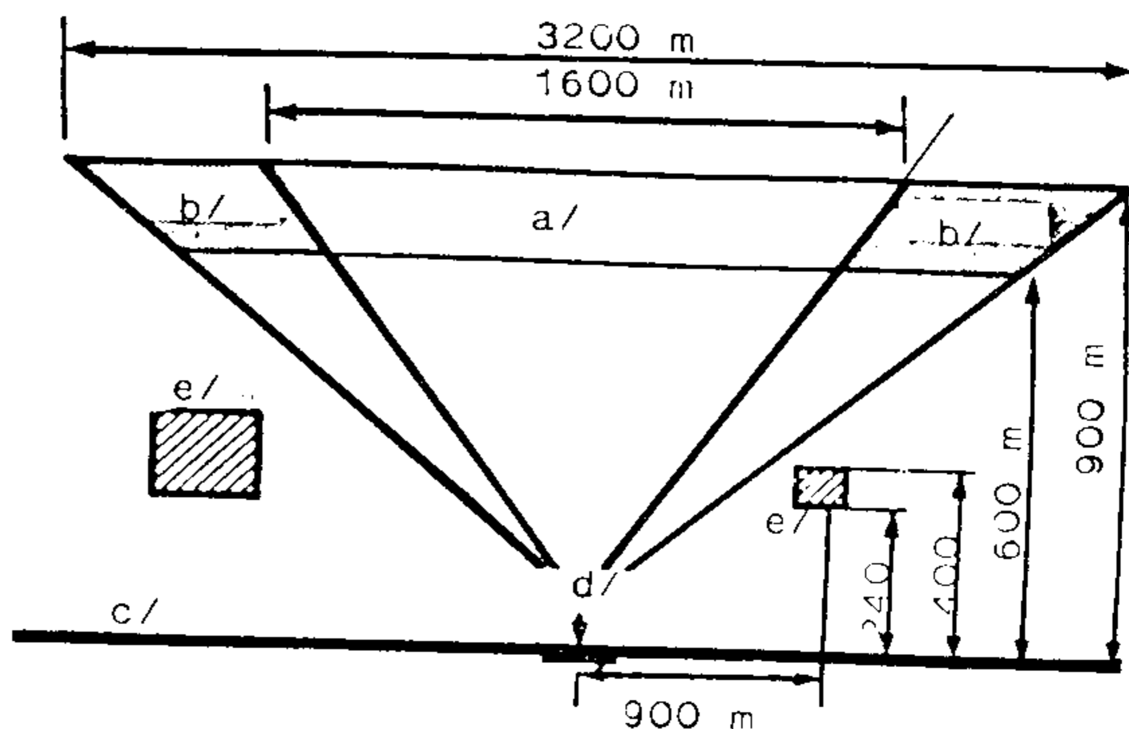
Ejtőernyős működési körzet metszete
